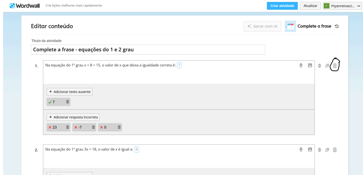
Figura 2 - Excluir conteúdo
